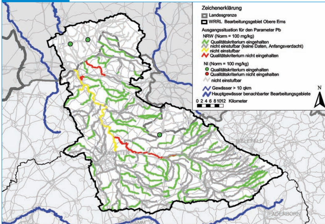
▶ Abb. 2.1.3.6-10 Ausgangssituation für den Parameter Blei
