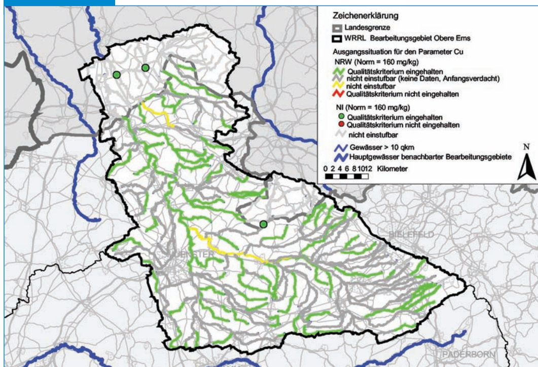
▶ Abb. 2.1.3.6-4 Ausgangssituation für den Parameter Kupfer
