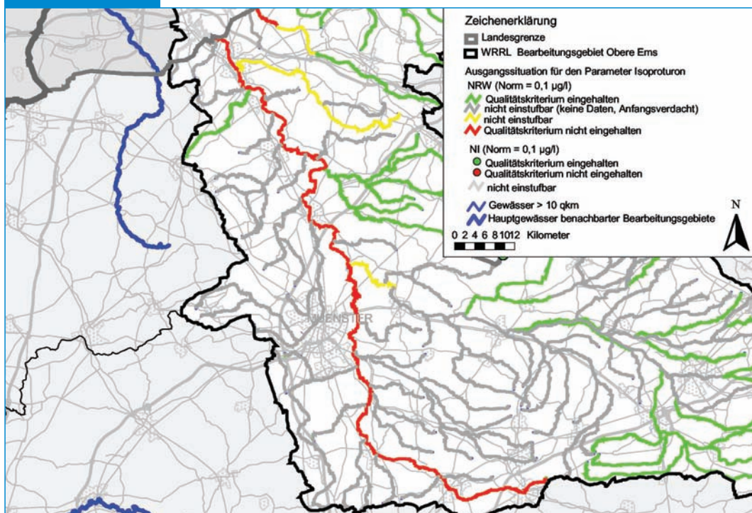
► Abb. 2.1.3.6-15 Belastungsschwerpunkte an der Werse (Beispiel Isoproturon)
