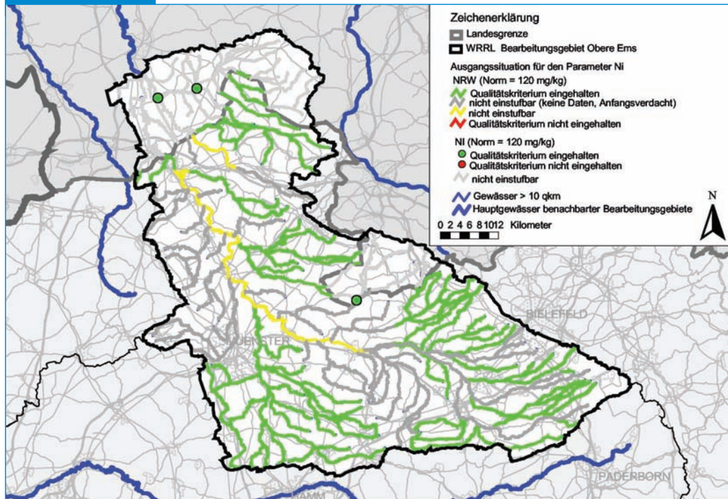
▶ Abb. 2.1.3.6-9 Ausgangssituation für den Parameter Nickel
