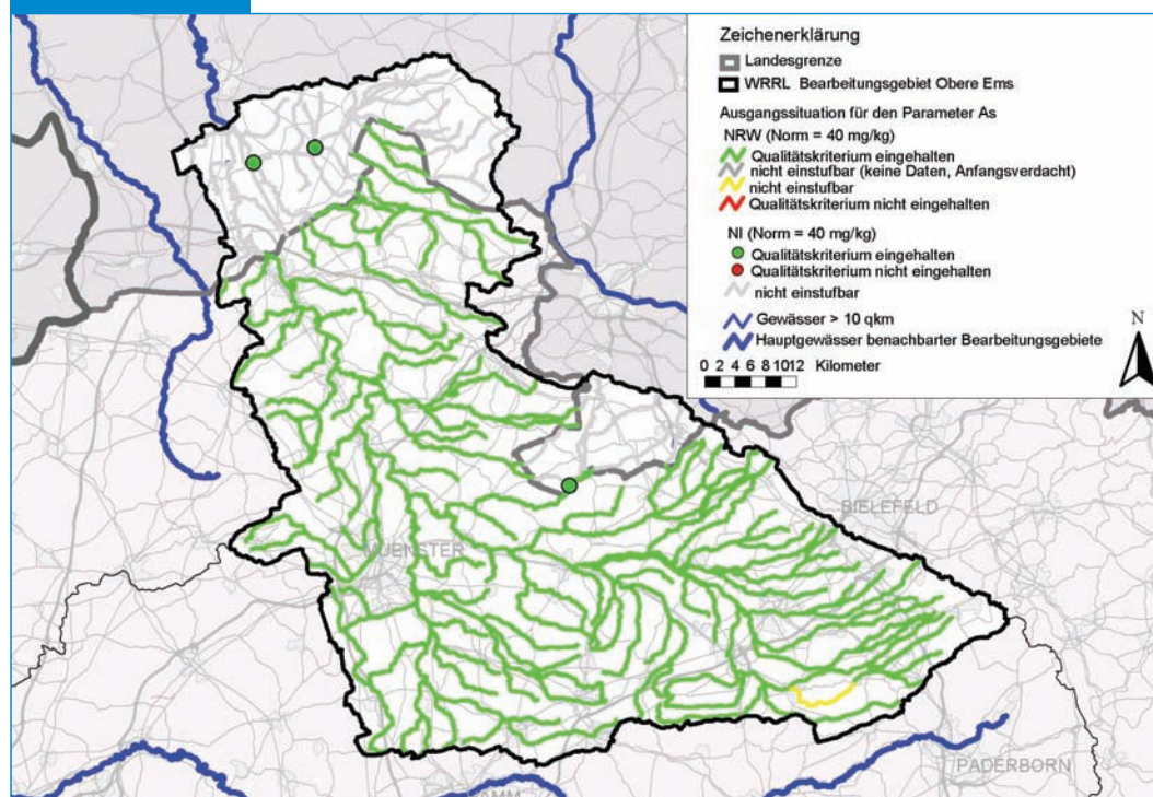
▶ Abb. 2.1.3.6-11 Ausgangssituation für den Parameter Arsen
