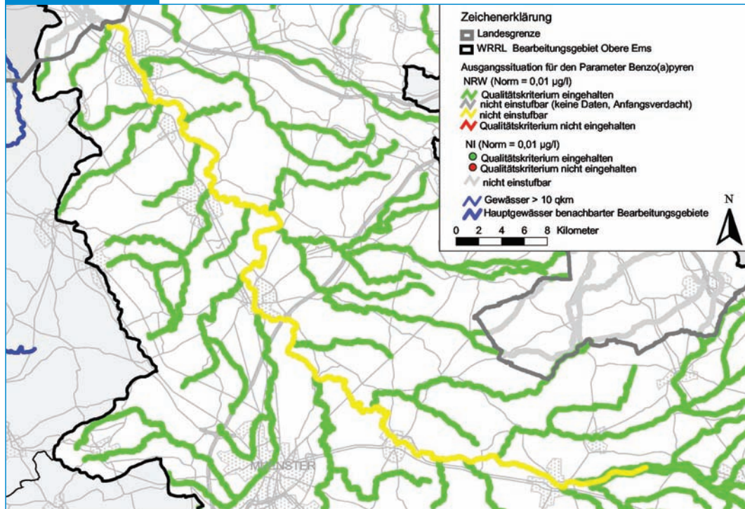
► Abb. 2.1.3.6-19 Belastung der Ems und der Bever mit PAK (Beispiel Benzo(a)pyren)
