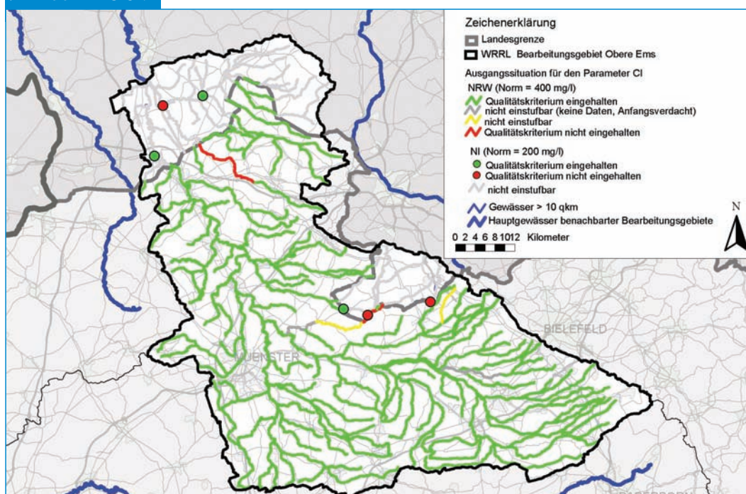
► Abb. 2.1.3.5-7 Ausgangssituation für den Parameter Chlorid
