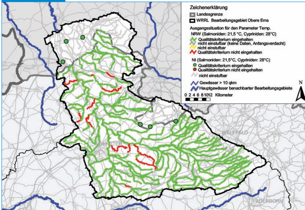
▶ Abb. 2.1.3.5-4 Ausgangssituation für den Parameter Temperatur
