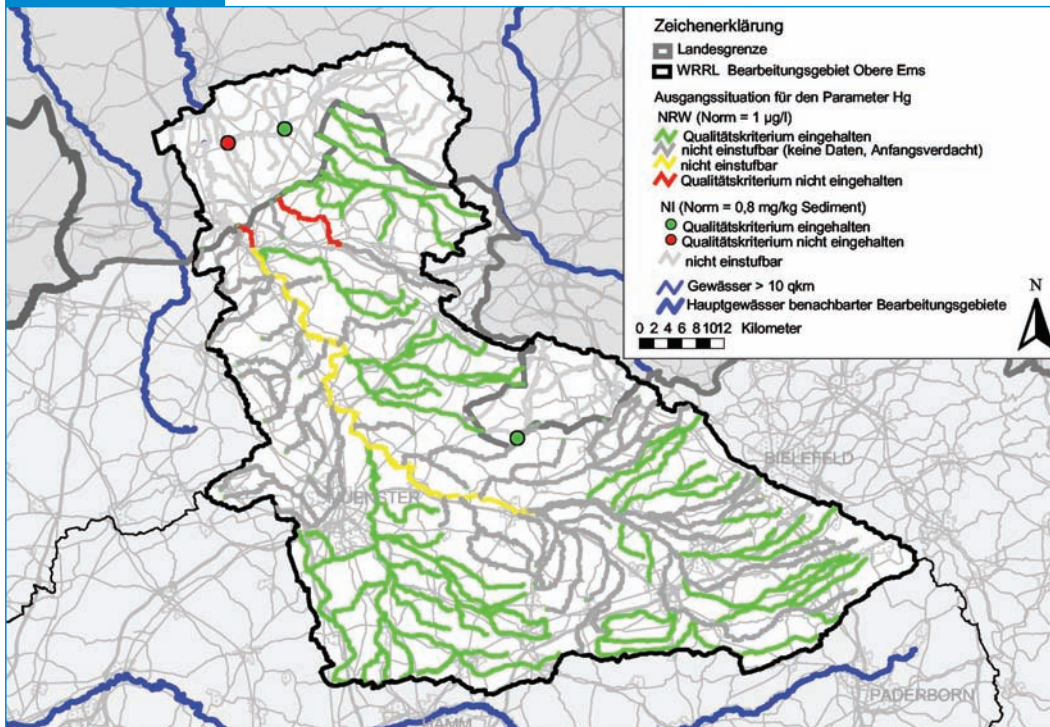
▶ Abb. 2.1.3.6-8 Ausgangssituation für den Parameter Quecksilber
