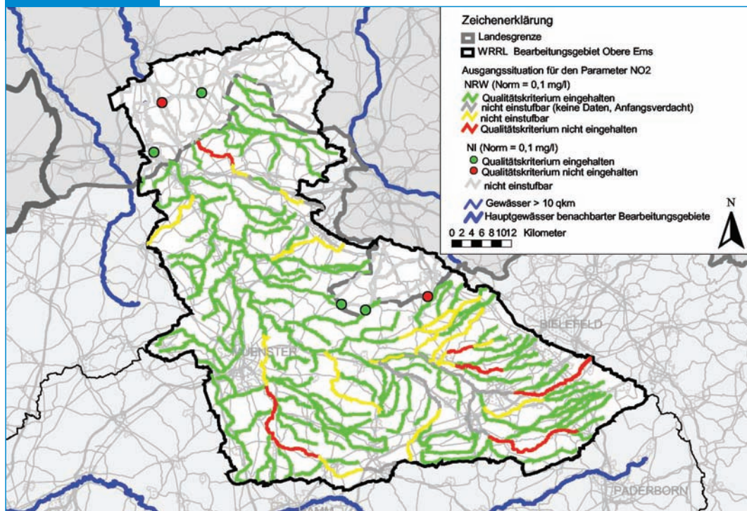
▶ Abb. 2.1.3.6-20 Ausgangssituation für den Parameter Nitrit
