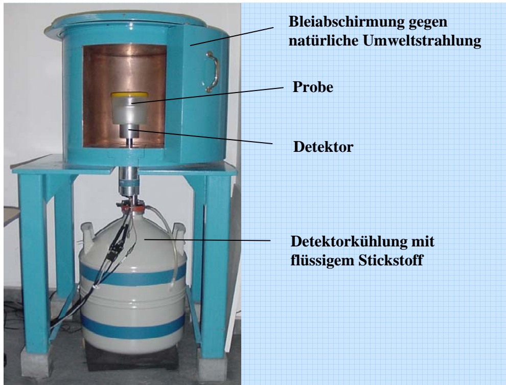
Abbildung 2.5: Messplatz für Gammaskopimetrie
