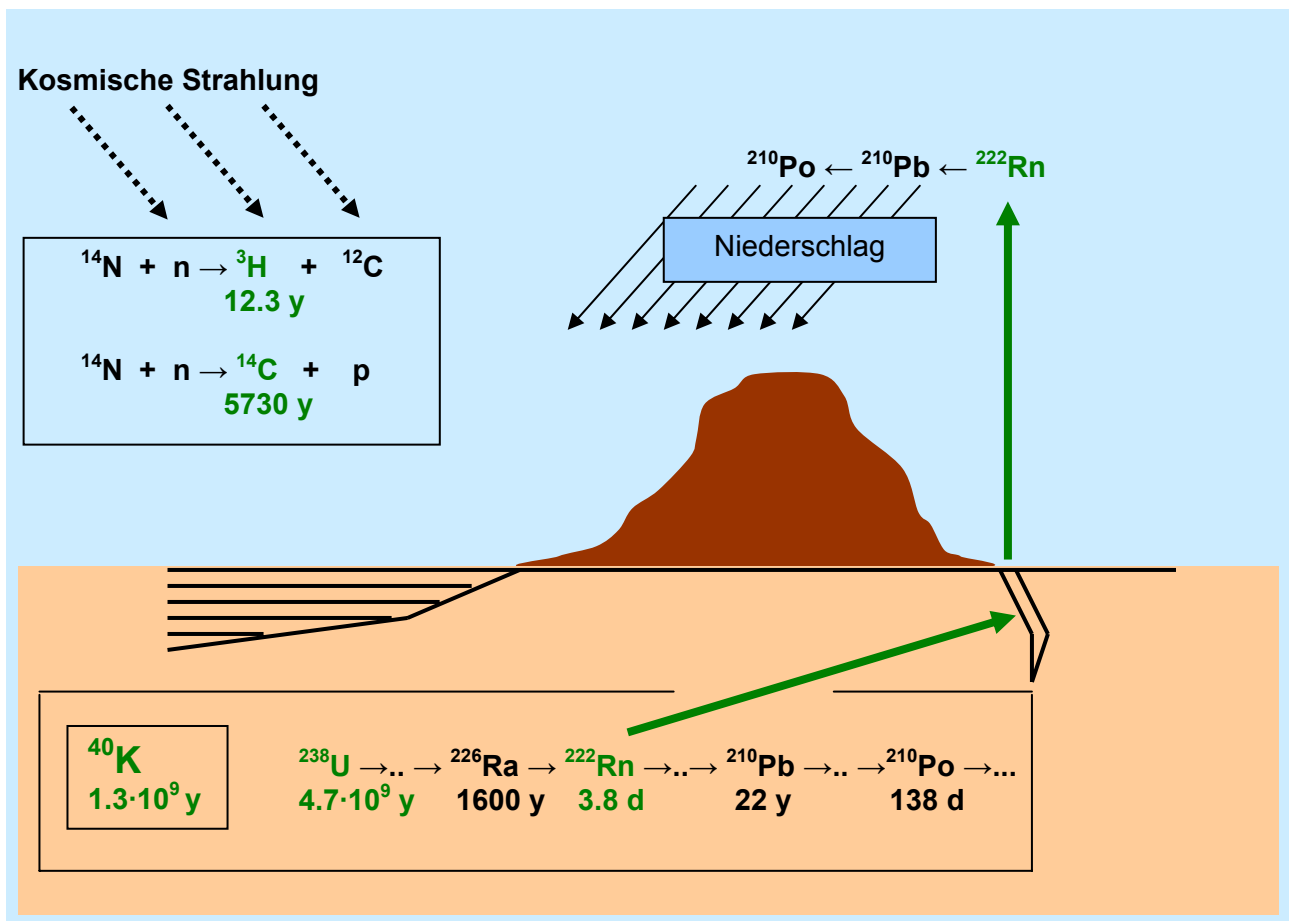
Abbildung 2.3: Natürliche radioaktive Stoffe in Atmosphäre und Boden und deren physikalische Halbwertszeiten (y = Jahre, d = Tage, 10 9 = 1 Milliarde)
