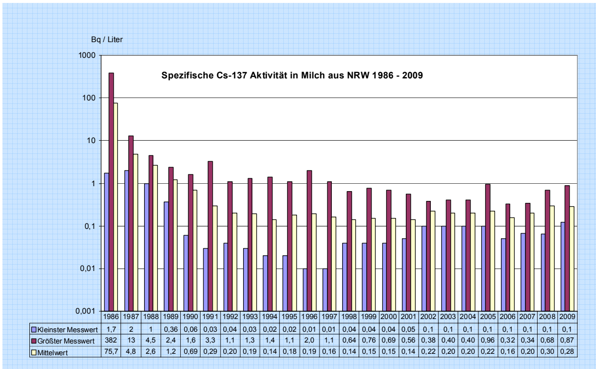
Abbildung 5.3: Spezifische Cs-137 Aktivität in Milch NRW 1986 - 2009
