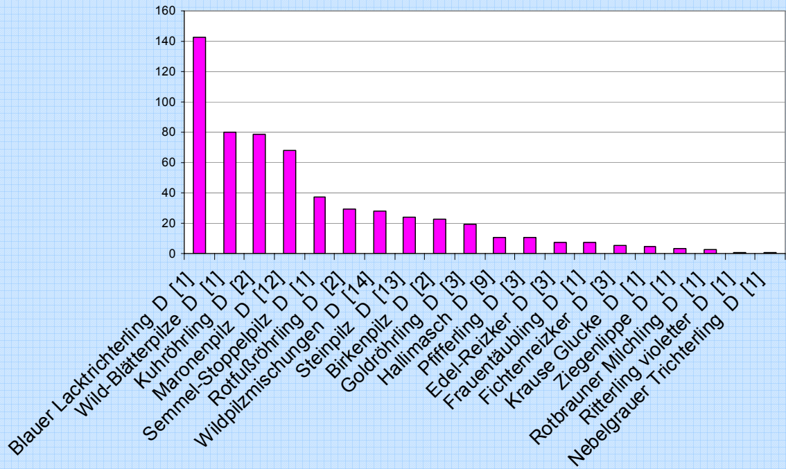
Abbildung 5.5 Spezifische Cs-137 Aktivität in Wildpilzen aus NRW 2009 Mittelwerte aus Einzelwerten bzw. Einzelwerte, Klammerangaben: Anzahl der Proben
