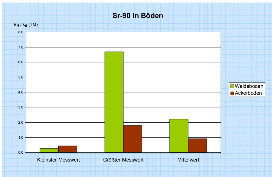
Abbildung 5.2: Spezifische Sr-90 Aktivität in verschiedenen Bodenarten NRW 2009
