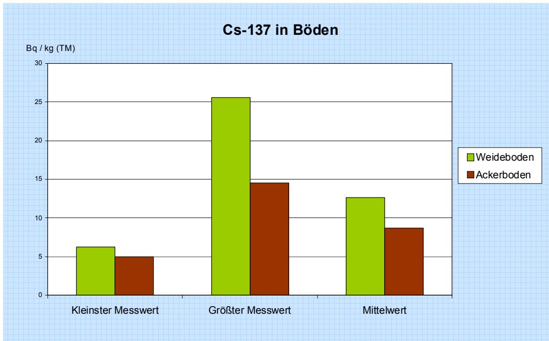
Abbildung 5.1: Spezifische Cs-137 Aktivität in verschiedenen Bodenarten NRW 2009
