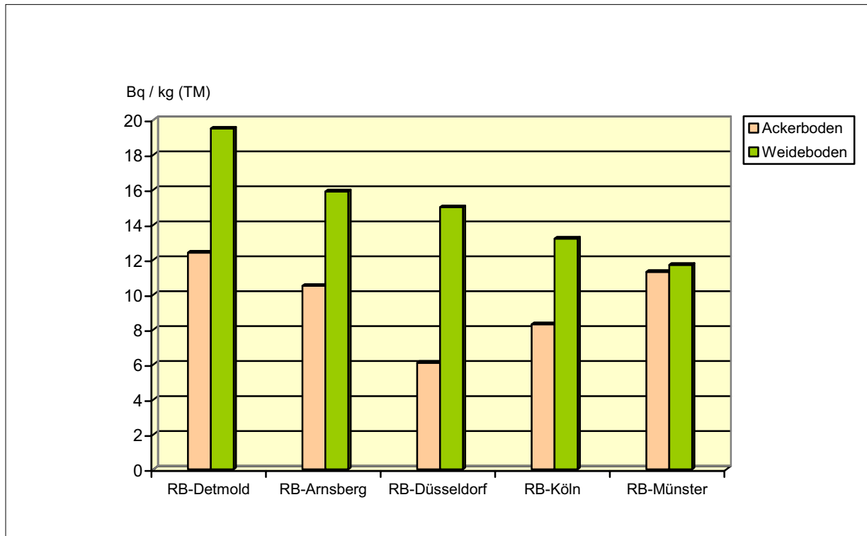
Abb. 5.2: Spezifische Cs-137 Aktivität im Boden NRW 2003 Mittelwerte auf Regierungsbezirksebene
