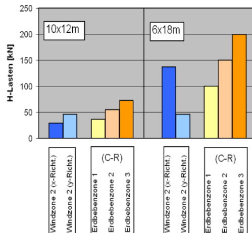
Bild 21 Vergleich der gesamten Windkraft mit der Gesamterdbebenkraft 2-geschossiger Holzhäuser
