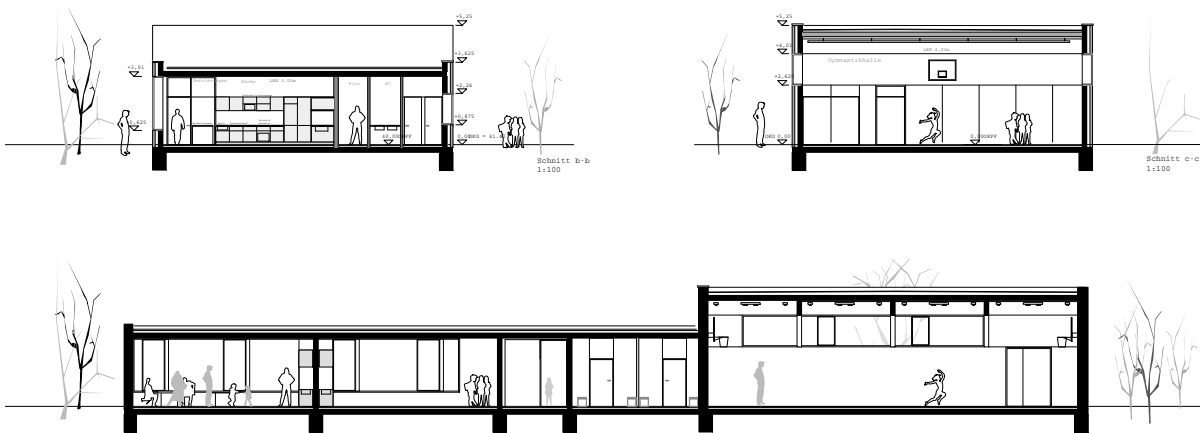
Schnitte
