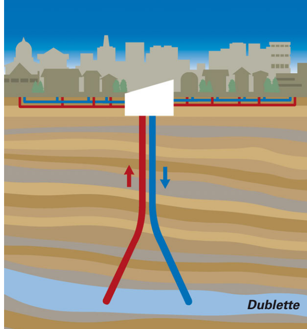
Tiefe Erdwärmesonde
