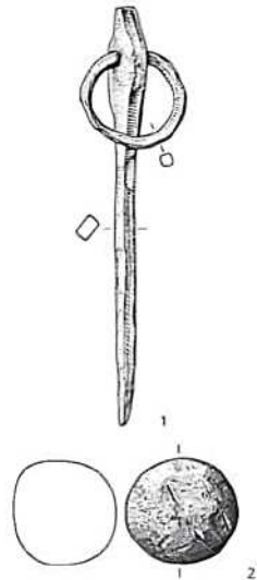
33 Neuss-Rosellen. Eiserner Zelthering (1) und Tonkugel (2) aus dem Bereich der Villa rustica. – Maßstab 1:2.
