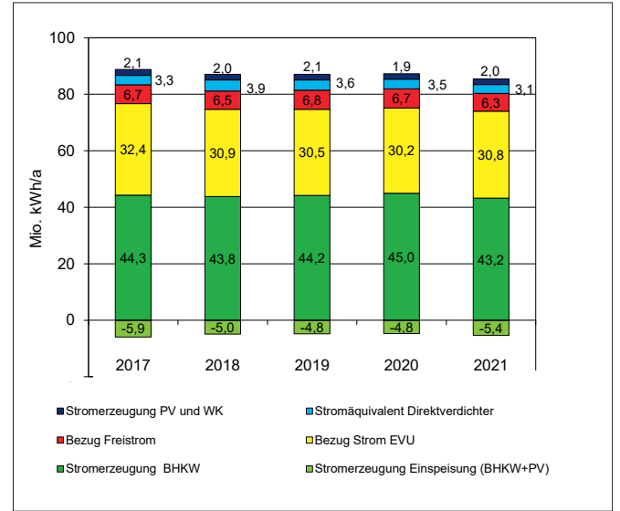
Bild 13.8: Energieeinsatz auf den Ruhrverbandskläranlagen von 2017 bis 2021 Fig. 13.8: Energy data from the Ruhrverband's sewage treatment plants from 2017 to 2021
