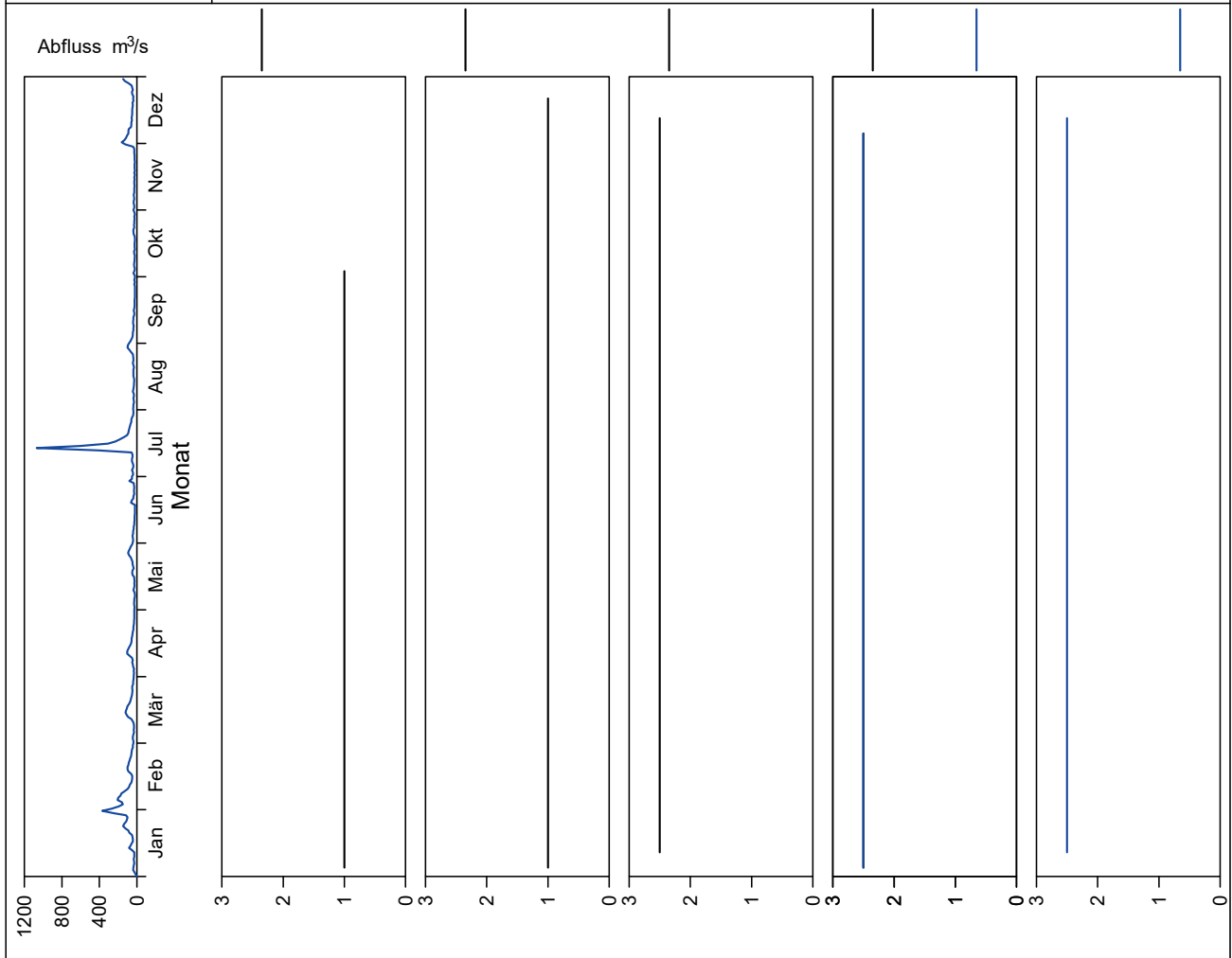
Bild 21.30: Analysenstatistik verschiedener Kenngrößen im Ruhrwasser Fig. 21.30: Statistics on the analysis of selected parameters in Ruhr water 8
