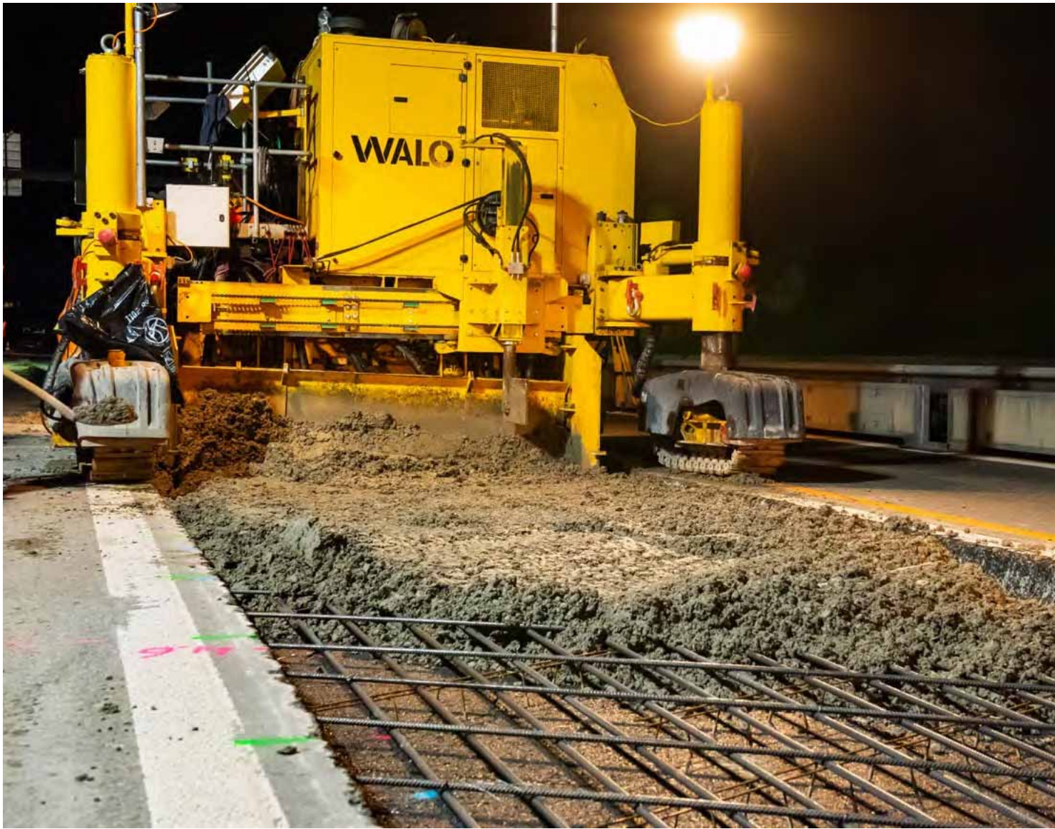
Maschineller Einbau mit Gleitschalungsfertiger
