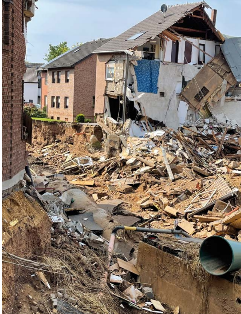
Erosionsrinne und Gebäudeschäden in der Ortslage Blessem nach dem Absinken des Wasserstandes in der Kiesgrube (27. Juli)
