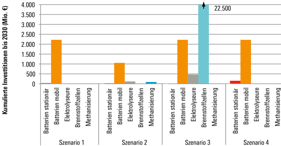
Kumulierte Investitionen der Szenarien 1 bis 4 (Zieljahr 2030) nach Technologien
