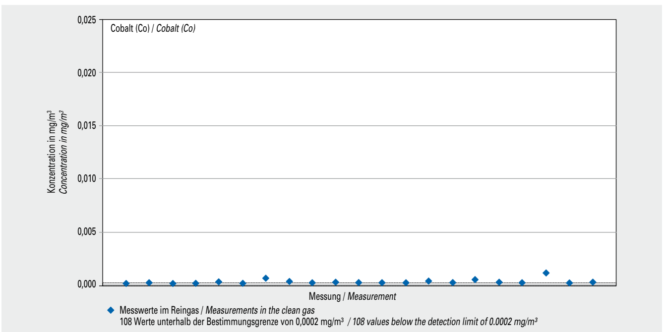
Bild 5-23 Messwerte (Jahr 2017) der Konzentration von Cobalt (Co) im Reingas von 39 Drehofenanlagen Fig. 5-23 Cobalt (Co) concentration values (year 2017) in the clean gas of 39 rotary kilns
