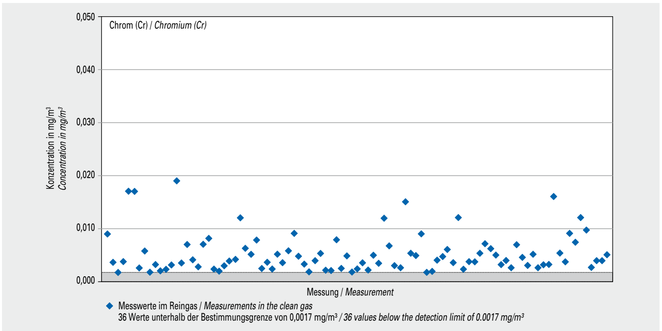
Bild 5-22 Messwerte (Jahr 2017) der Konzentration von Chrom (Cr) im Reingas von 39 Drehofenanlagen Fig. 5-22 Chromium (Cr) concentration values (year 2017) measured in the clean gas of 39 rotary kilns
