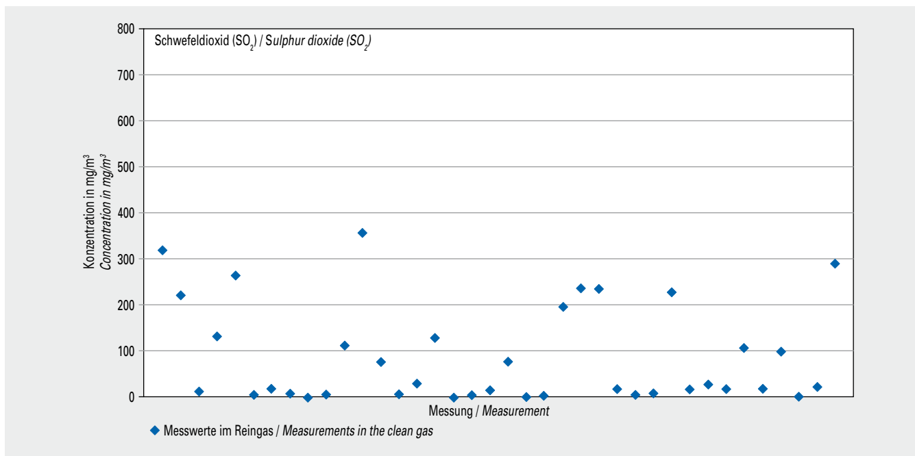
Bild 5-5 Mittelwerte (Jahr 2017) der Konzentration von Schwefeldioxid (SO 2 ) im Reingas von 38 Drehofenanlagen Fig. 5-5 Average sulphur dioxide (SO 2 ) concentration values (year 2017) measured in the clean gas of 38 rotary kilns
