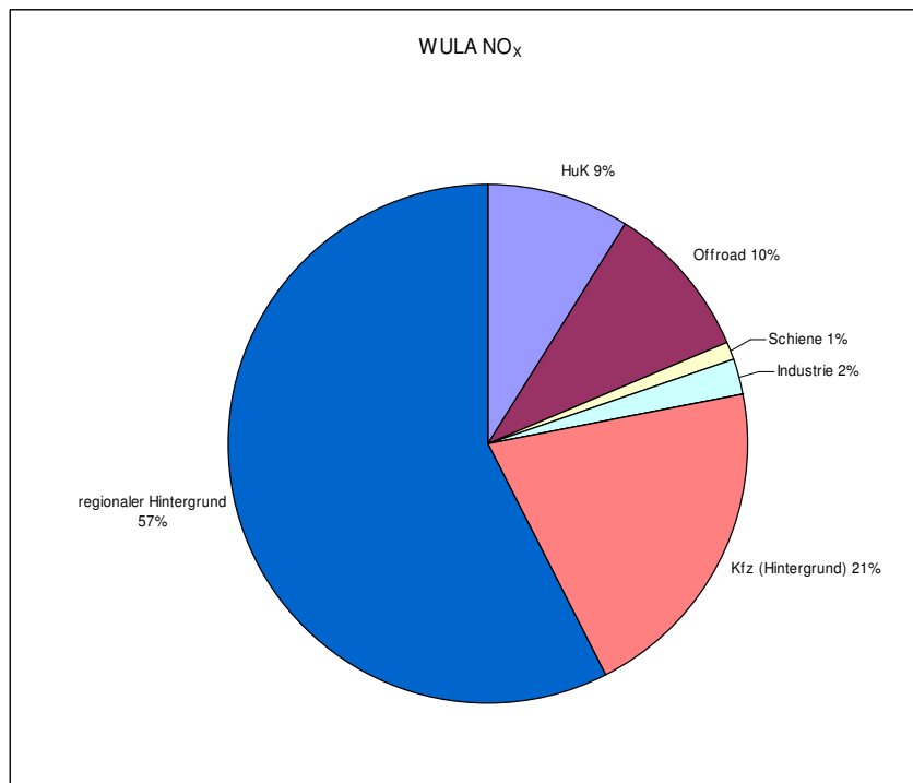
Abb. 3.3/6: Berechnete \text{NO}_x - Immissionsbeiträge nach Quellgruppen in % am Ort der Messstation WULA
