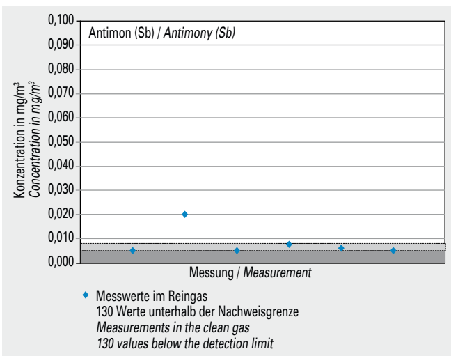
Bild 5-31 Messwerte (Jahr 2013) der Konzentration von Antimon (Sb) im Reingas von 38 Drehofenanlagen. Fig. 5-31 Antimony (Sb) concentration values (year 2013) measured in the clean gas of 38 rotary kilns.
