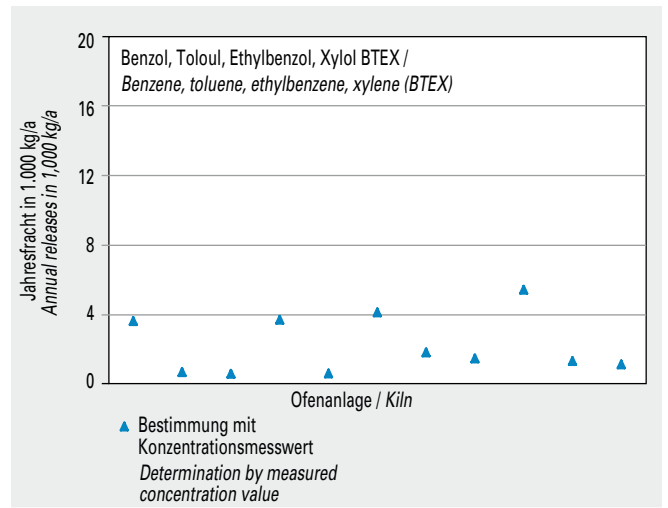
Bild 5-18 Emissionen von Benzol, Toluol, Ethylbenzol, Xylol (BTEX) von 11 Drehofenanlagen (Jahresfracht 2013). Fig. 5-18 Benzene, Toluene, ethylbenzene, xylene (BTEX) emissions (annual releases in 2013) of 11 rotary kilns.
