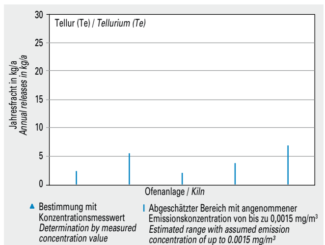
Bild 5-56 Emissionen von Tellur (Te) von fünf Drehofenanlagen (Jahresfracht 2013).
