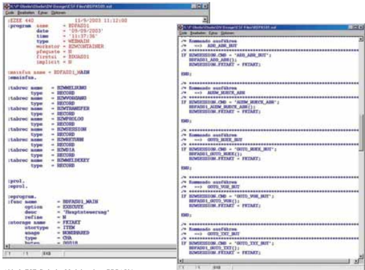
Abb. 9: ESF-Code der Modulstruktur BDPAS01
