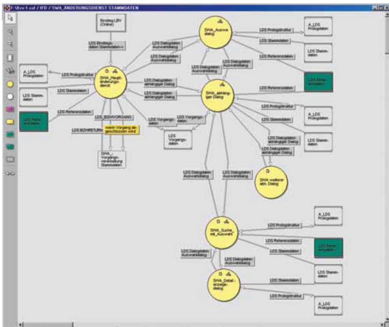
Abb. 1: SW-Architektur Änderungsdienst Stammdaten
