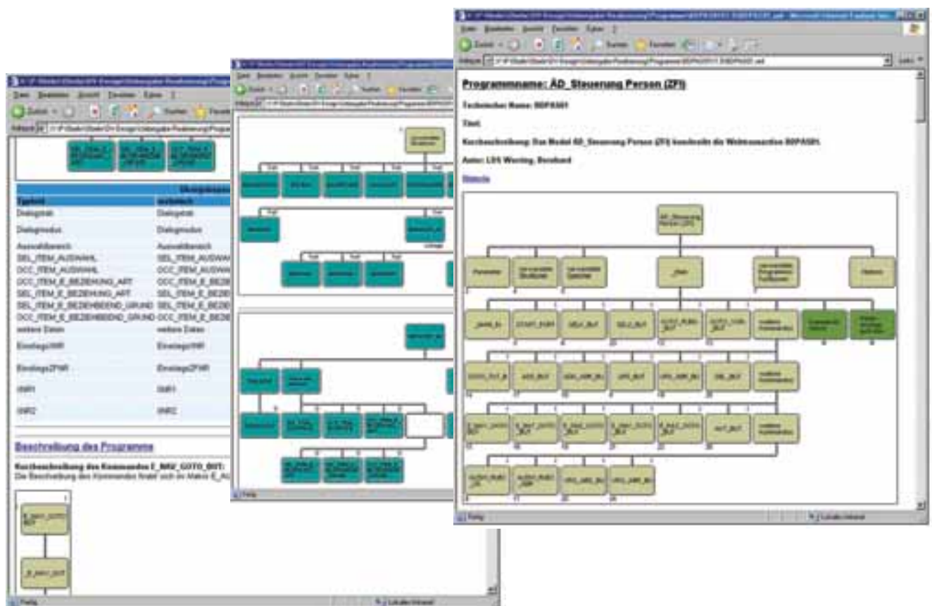
Abb. 10: XML-Programmvorgabe
