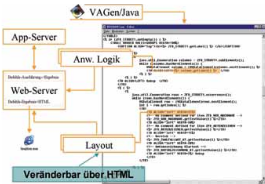
Abb. 14: JSP-File manipulieren
